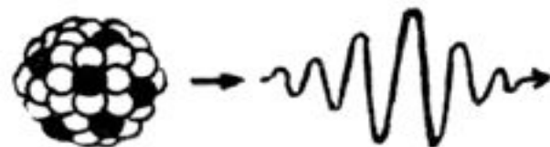
Гамма-квант
