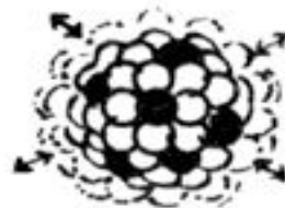
Возбуждённое ядро
