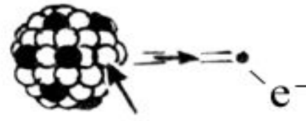
Протон
