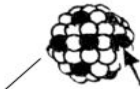
Ядро атома
