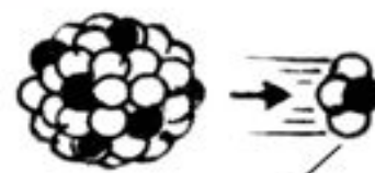
Альфа-частица
