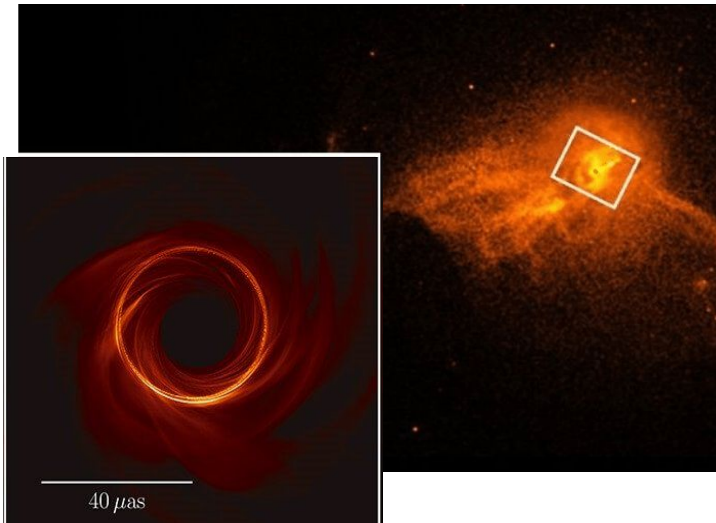
Снимок черной дыры 2019
