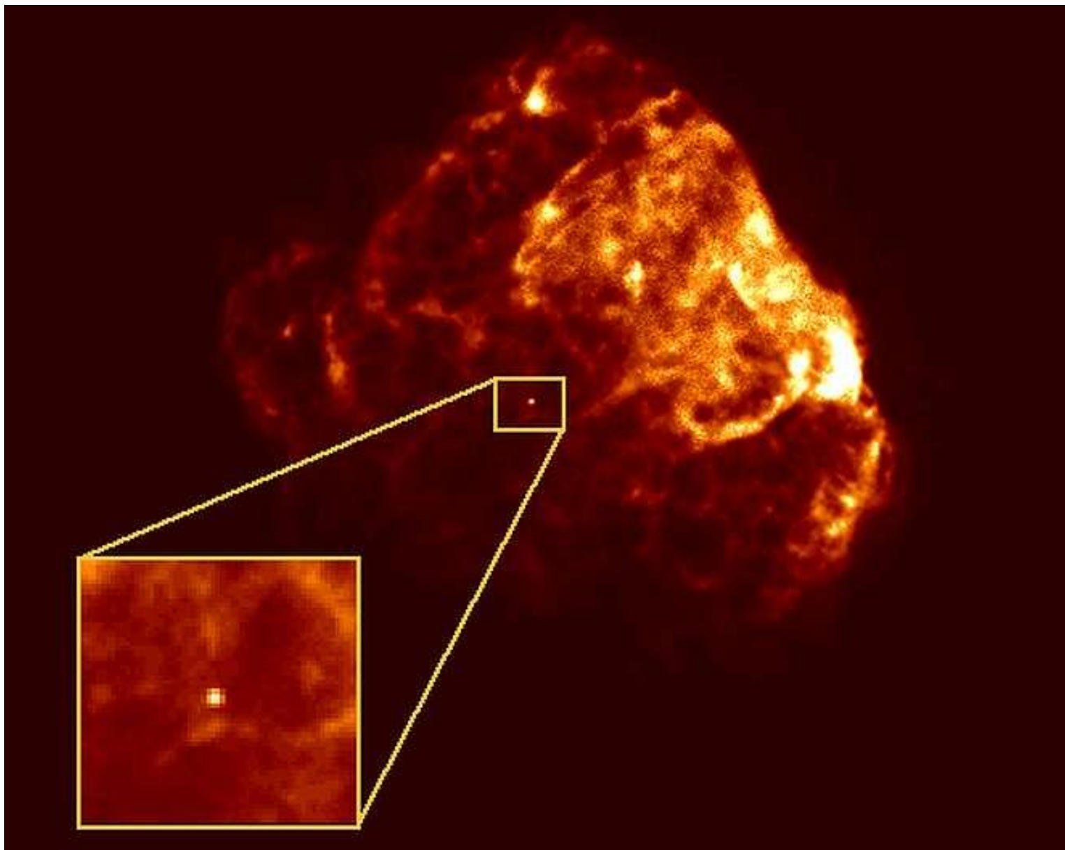
Остаток сверхновой Корма-А, в центре которой находится нейтронная звезда.
