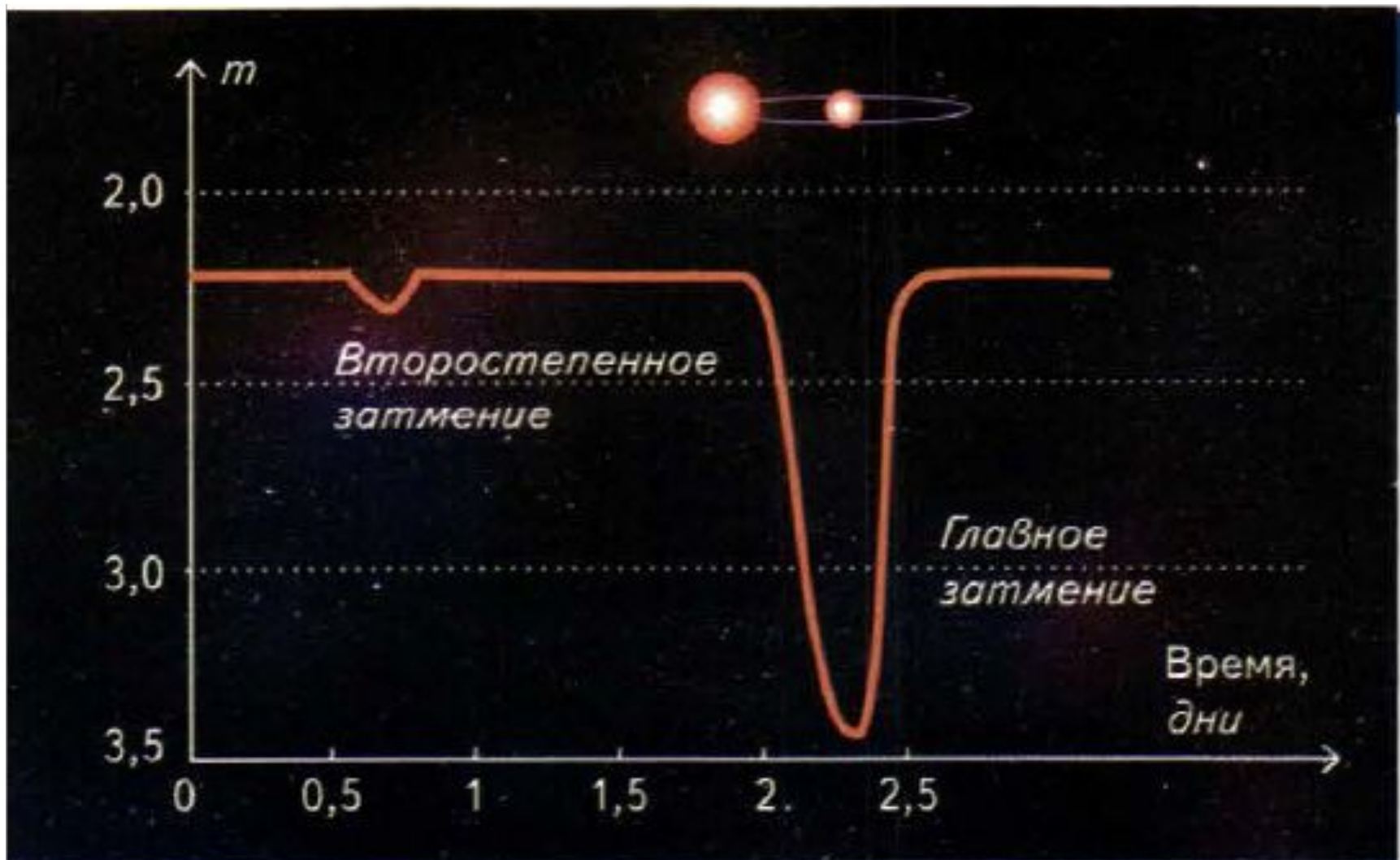
Зависимость звёздной величины от времени для затменно-переменной звезды
