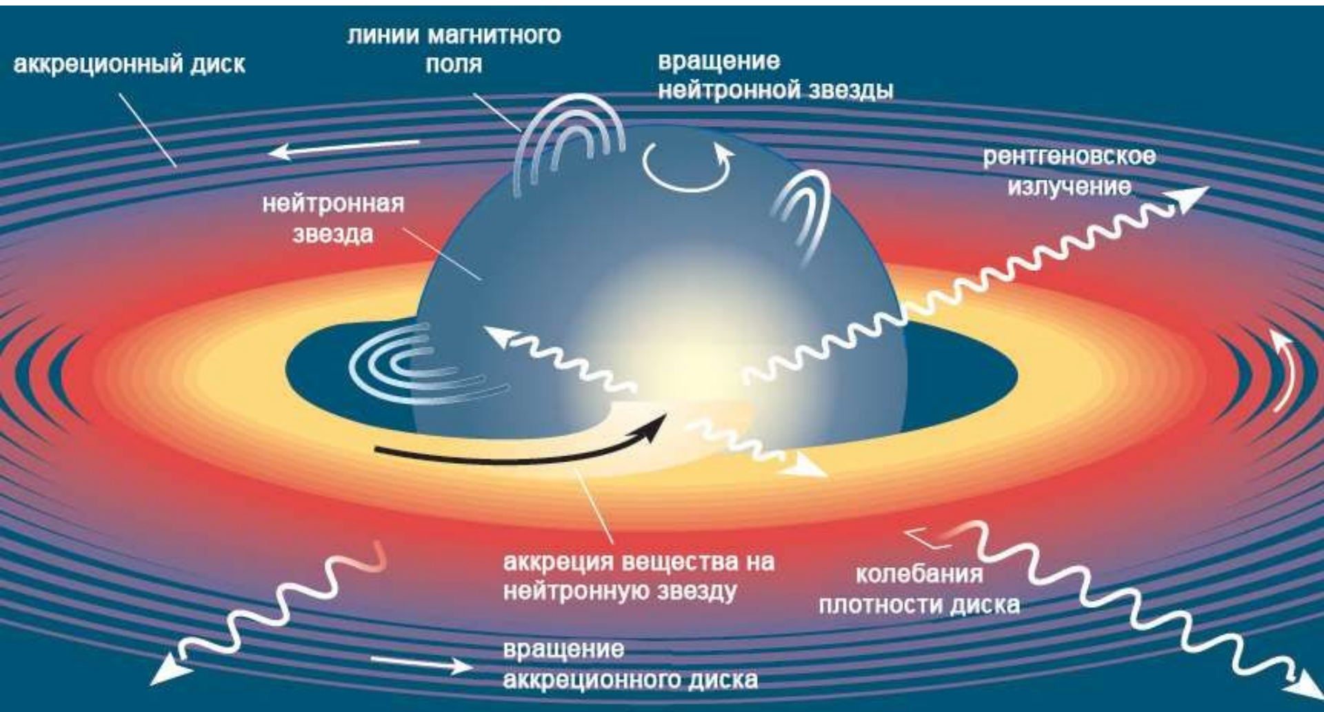
Акцерирующая нейтронная звезда
