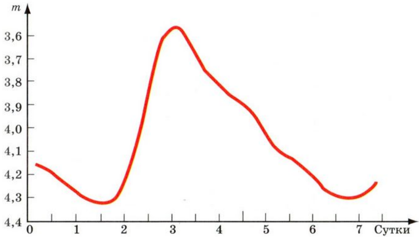
Рис. 92. Кривая блеска \delta Цефея
