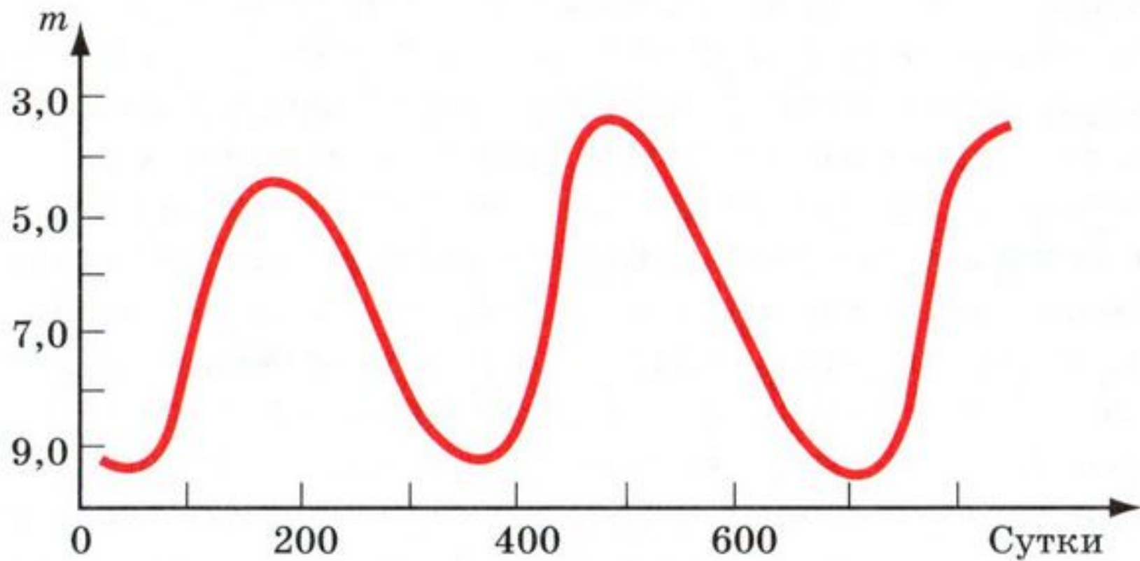
Рис. 94. Кривая блеска Миры Кита
