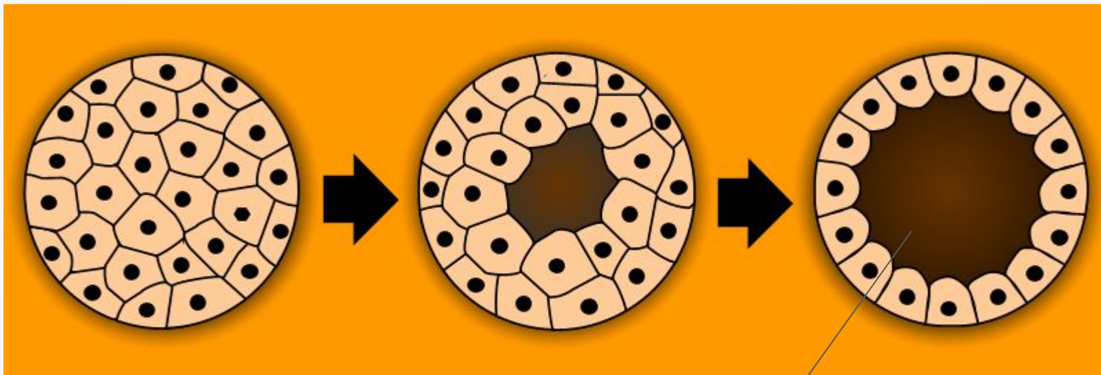
Бластула
