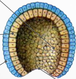
Гаструл а
