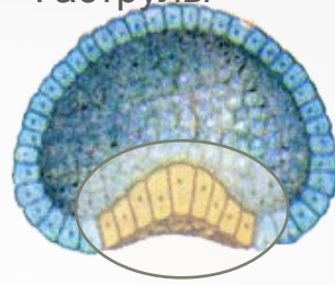
Образование Гастролы
