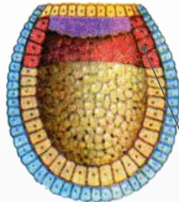
Ранняя нейрула
