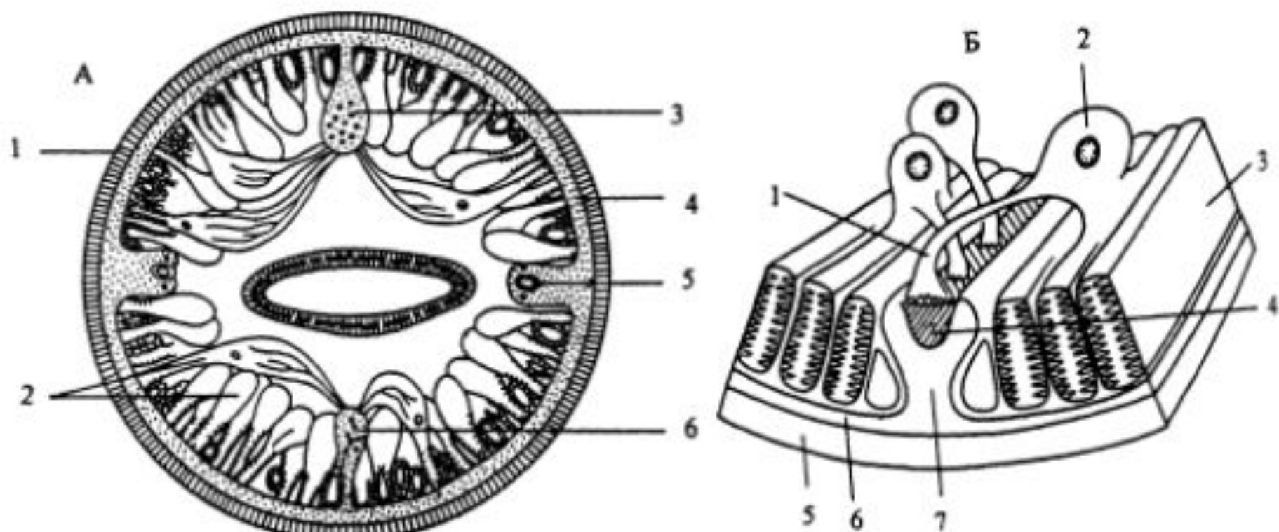
Рис. 5. Схема поперечного среза тела нематоды (А – Hartwich, 1993; Б – Барнс и др., 1992):
