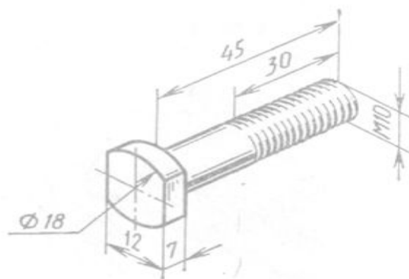
Винт
