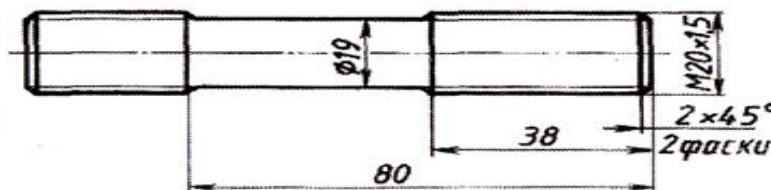
Шпилька ГОСТ 22032-76
