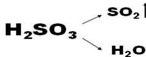
Сернистая кислота
