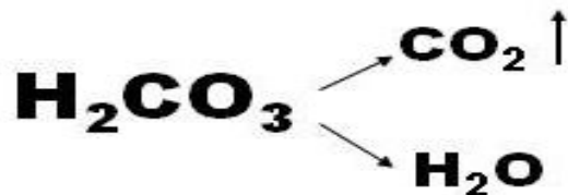
Угольная кислота
