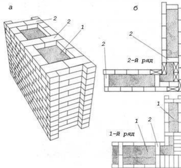
Рис. 5. «Колодцевая» кладка: а- фрагмент кладки; б- порядковая раскладка кирпичей при кладке прямого угла стены; 1- утеплитель; 2- диафрагма из тычковых кирпичей.
