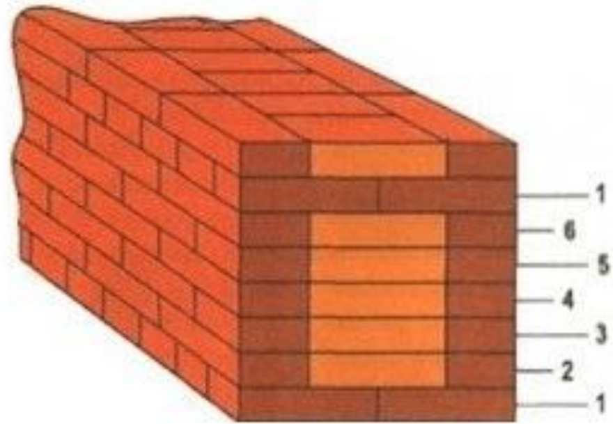
Рис.2 Многорядная система перевязки 1 - тычковый ряд; 2-6 - ложковые ряды
