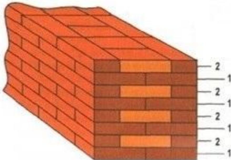
Рис.1 Двухрядная система перевязки 1 - тычковый ряд; 2 - ложковый ряд
