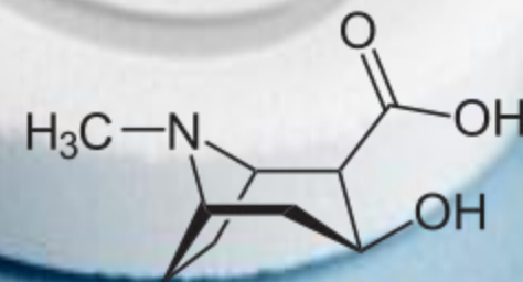
Экгонин
