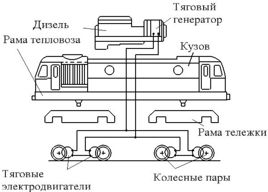
Рис. 1. Схема электрической передачи тепловоза
