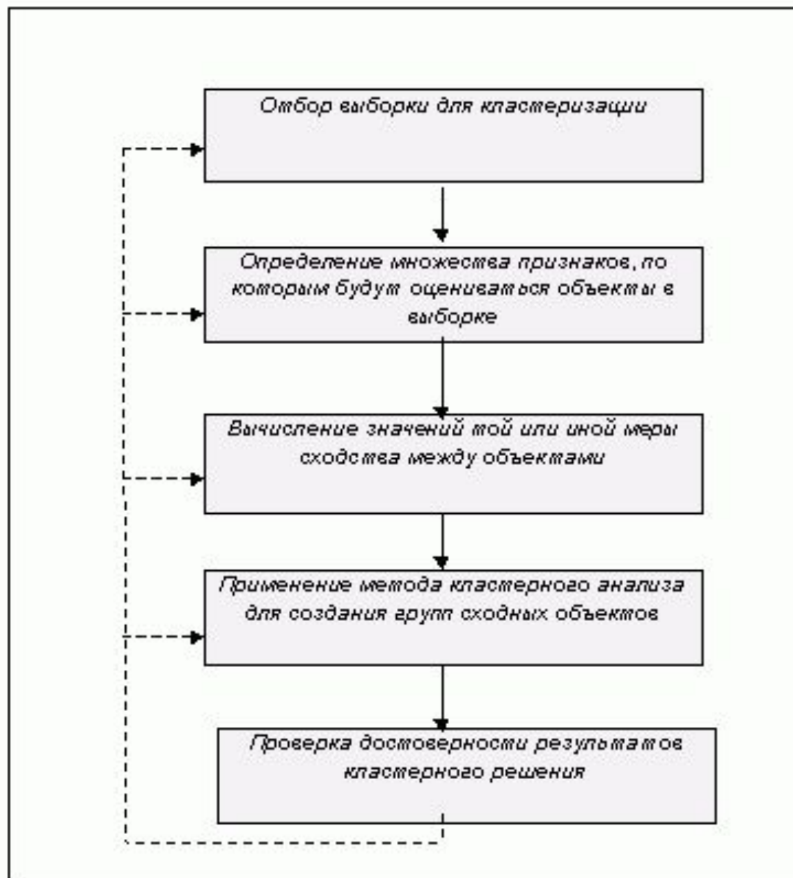
Рис. 1 Схема организации проведения кластерного анализа.
