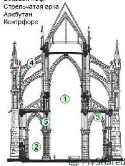
Конструкция готического храма
