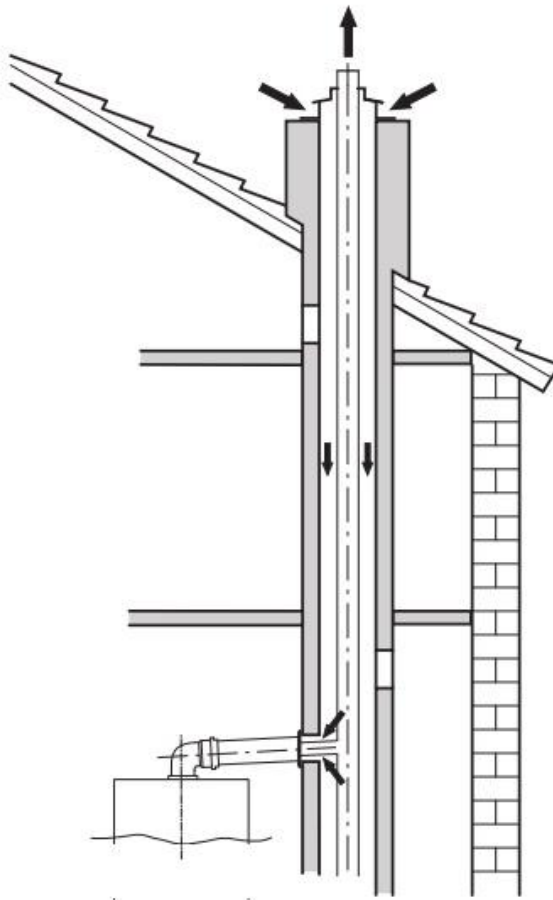
Рис. Концентрическое дымоотведение по C42x/C43x
