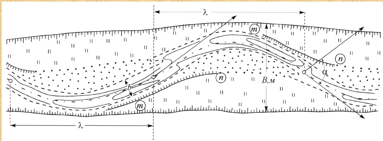
Схема ограниченного меандрирования.
