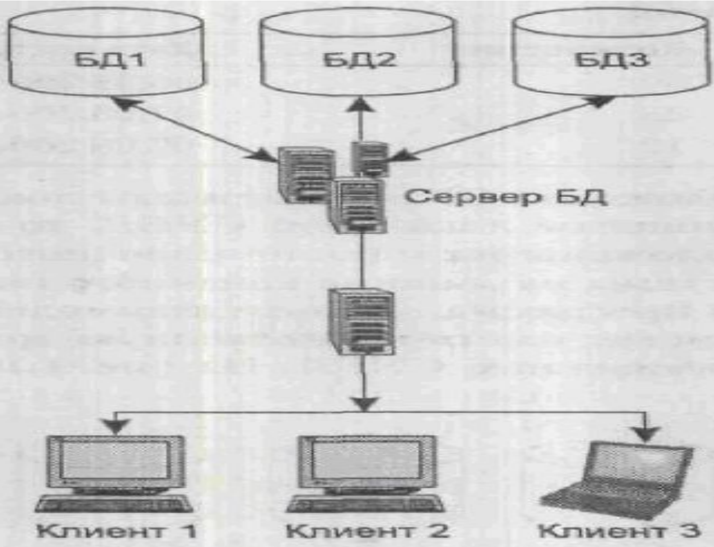
Рис. 1.2. Схема трехзвенной СУБД
