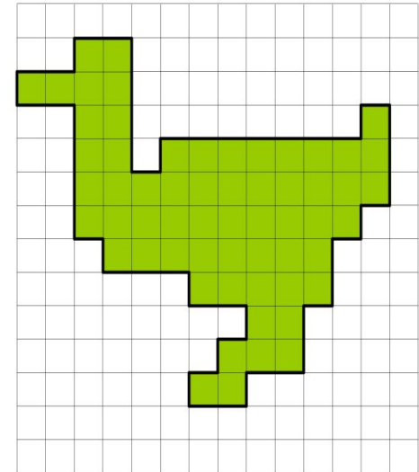
Pentomino Утка
