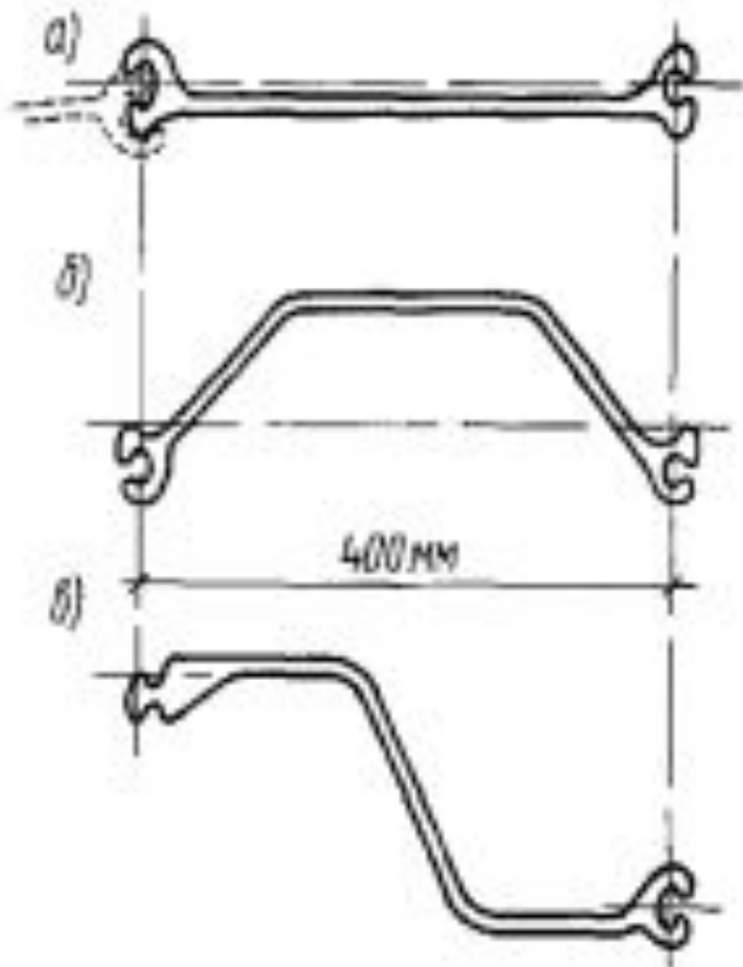
Рис. 14.4. Профили прокатного стального шпунта:
