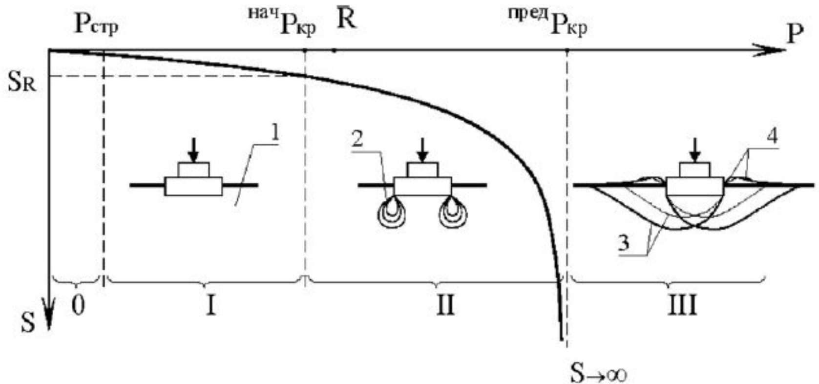
Рис. 4.1. Фазы напряженно-деформированного состояния грунта:
