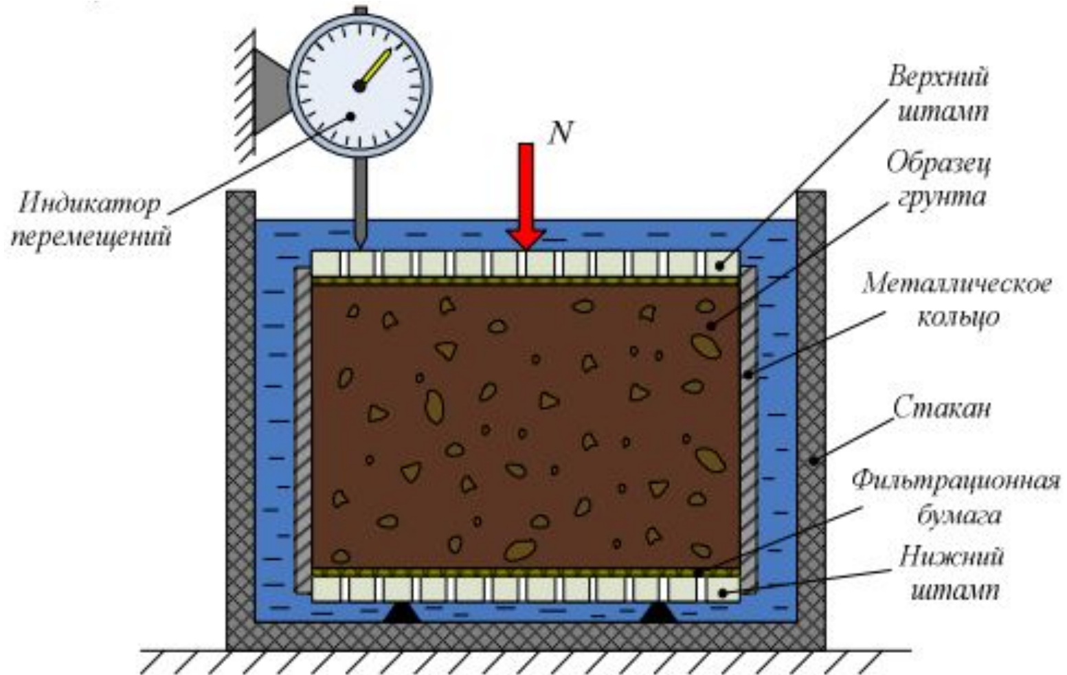
Рис.1. Общий вид компрессионного прибора -а), принципиальная схема прибора -б)
