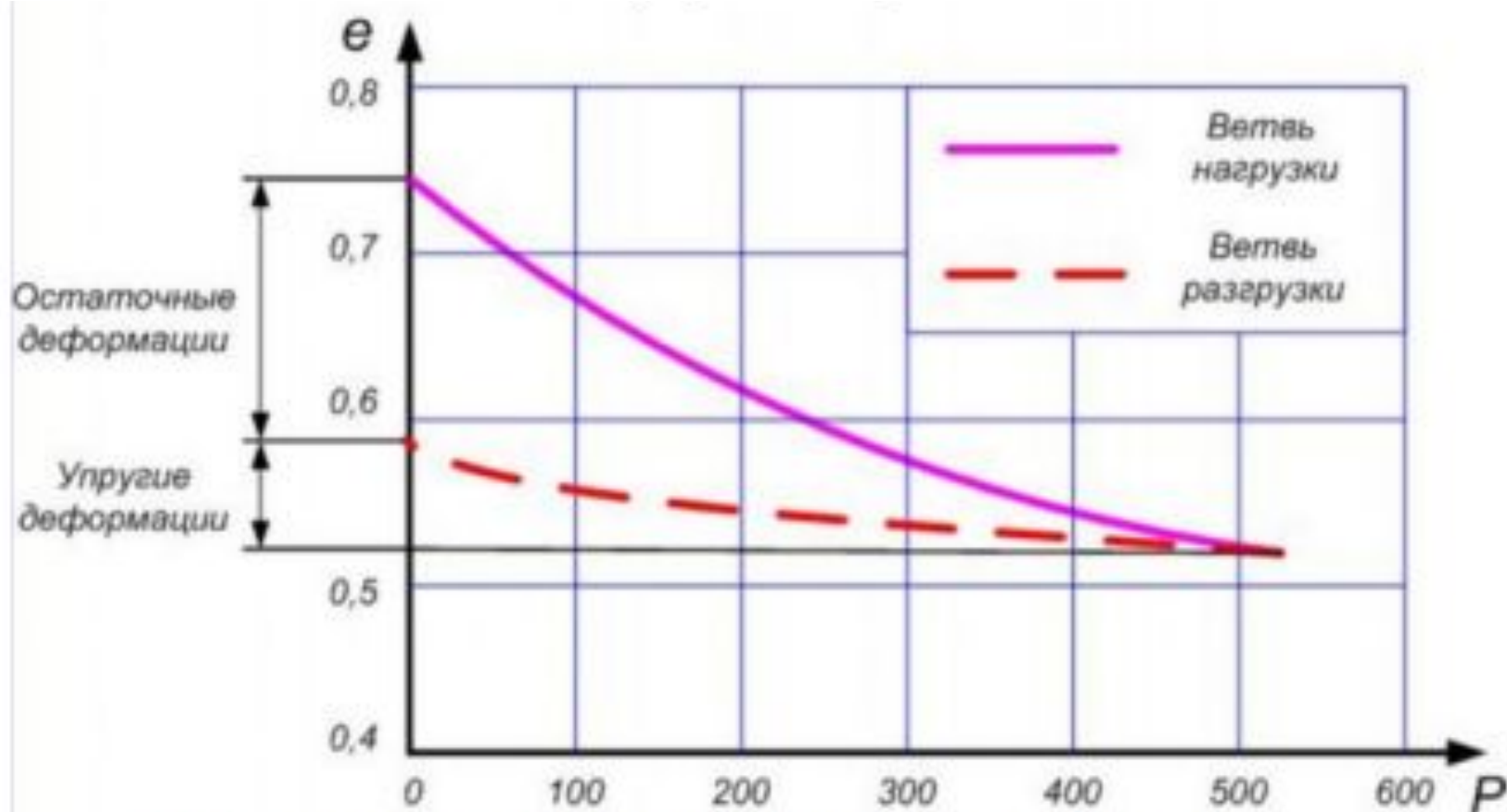
Рис.3. Общий вид компрессионной кривой
