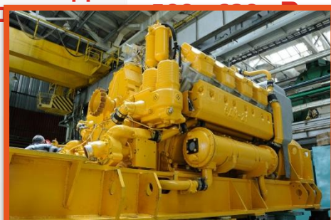
АДГ-1000 8-цилиндровый дизельный генератор. 1000 кВт
