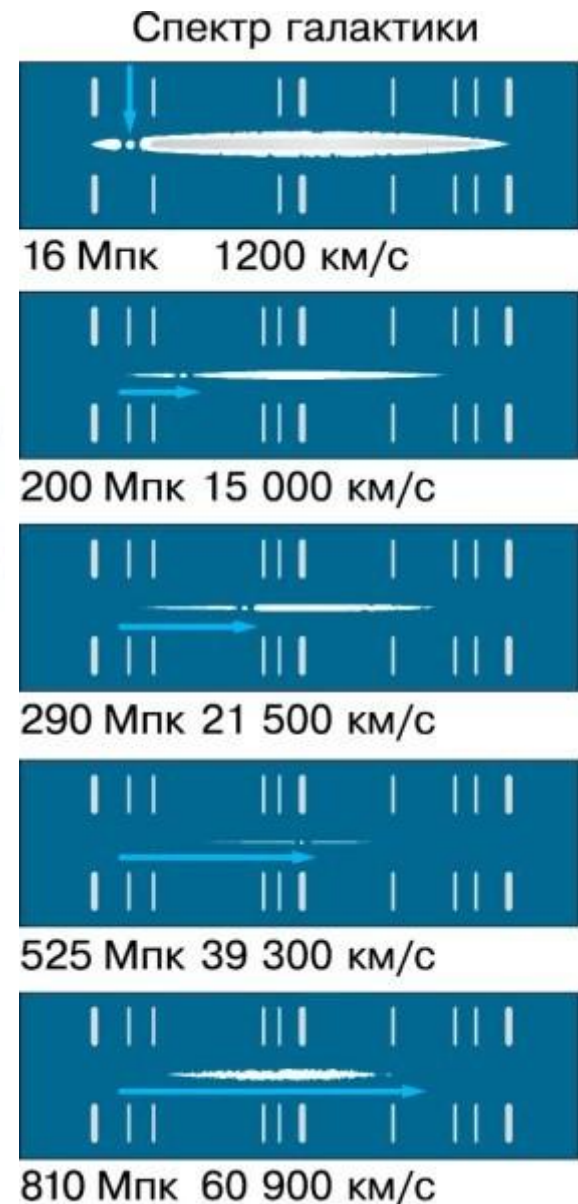
«Красное смещение» в спектрах галактик
