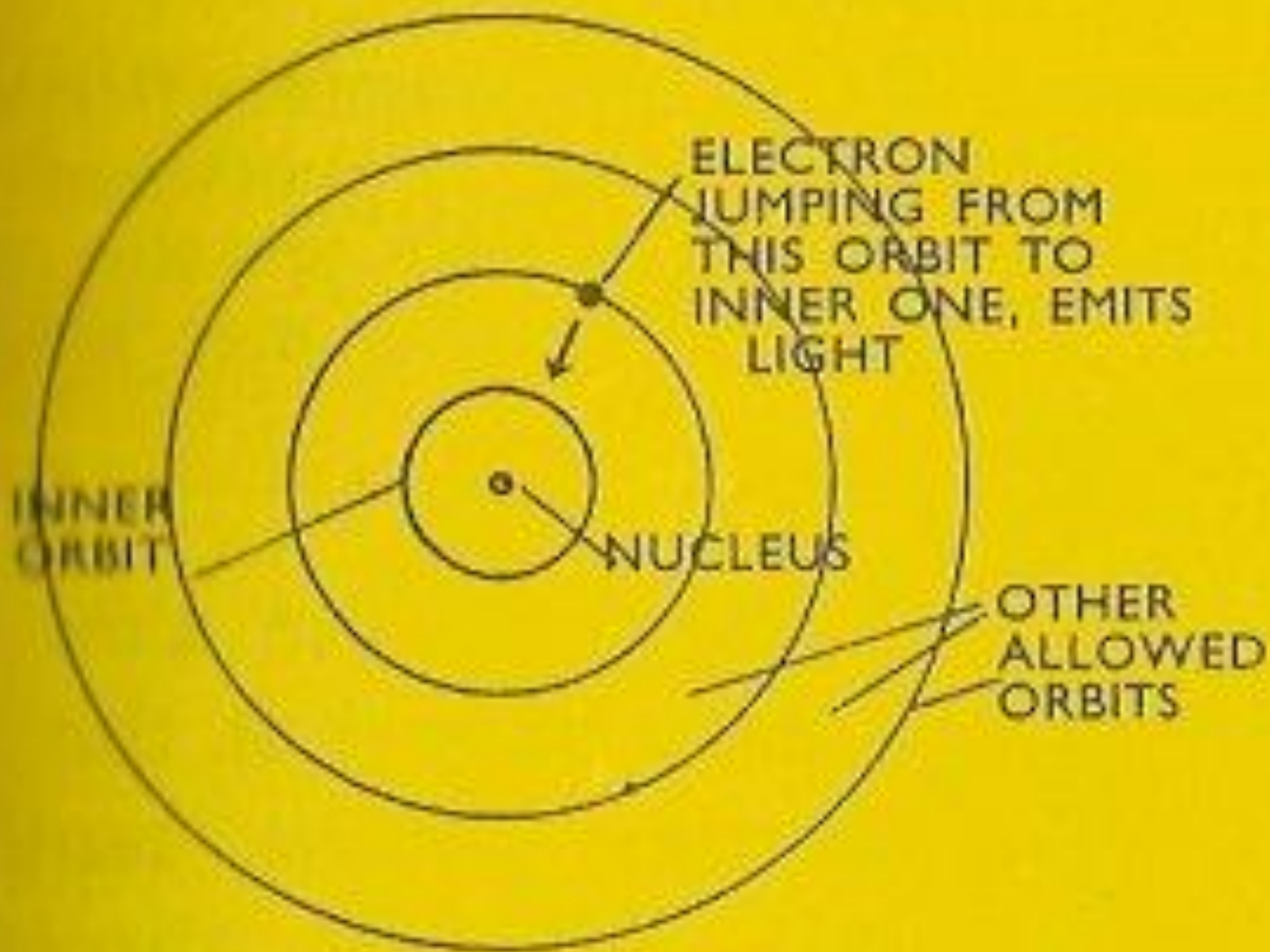
Bohr atom
