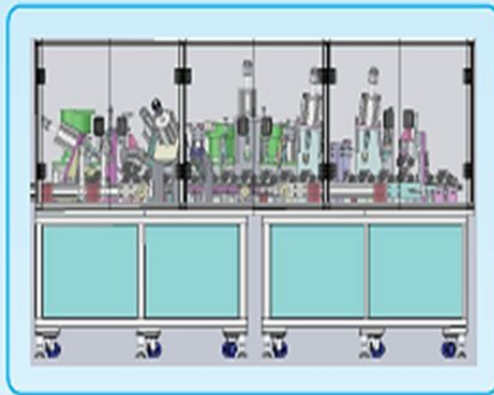
汽车、摩托车化油器组装生产线
