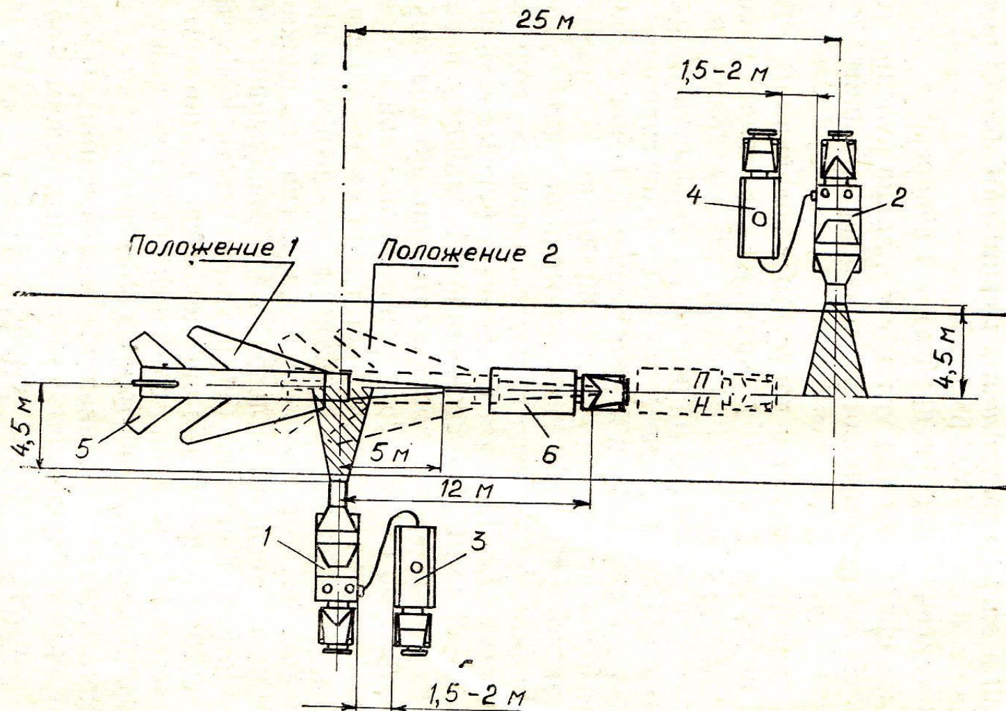
Рис. 3. Схема обработки самолета с помощью двух тепловых машин типа ТМС-65:
