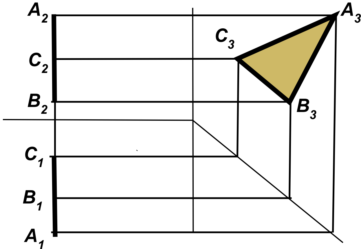
Чертеж профильной плоскости уровня
