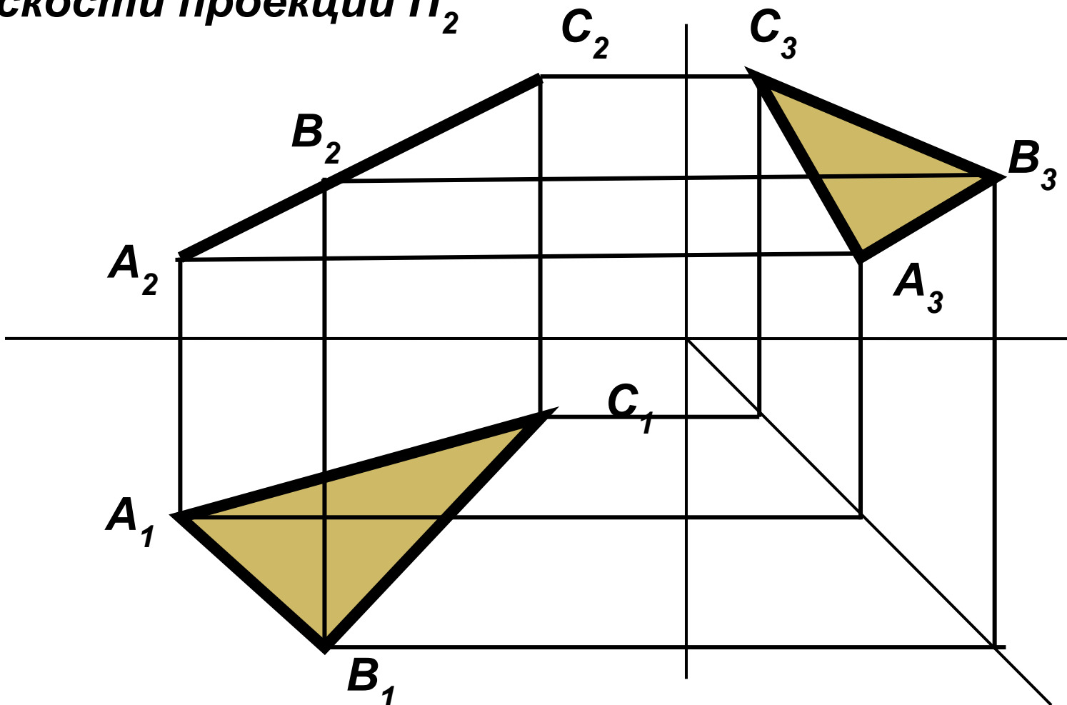
Чертеж фронтально-проецирующей плоскости
