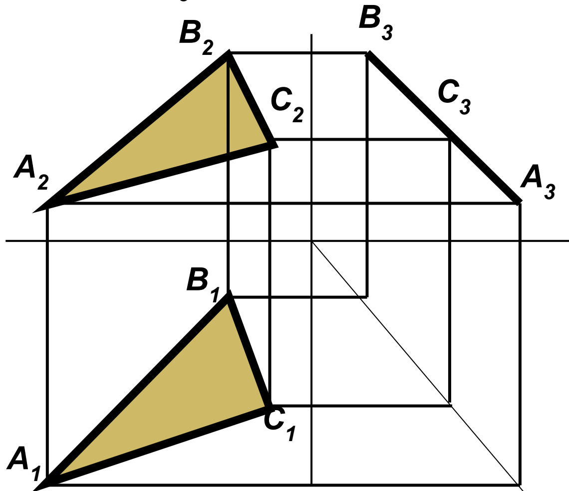
Чертеж профильно-проецирующей плоскости
