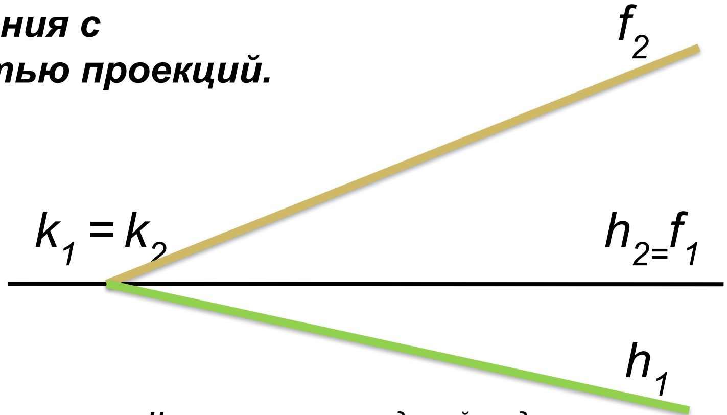
Чертеж плоскости заданной следами
