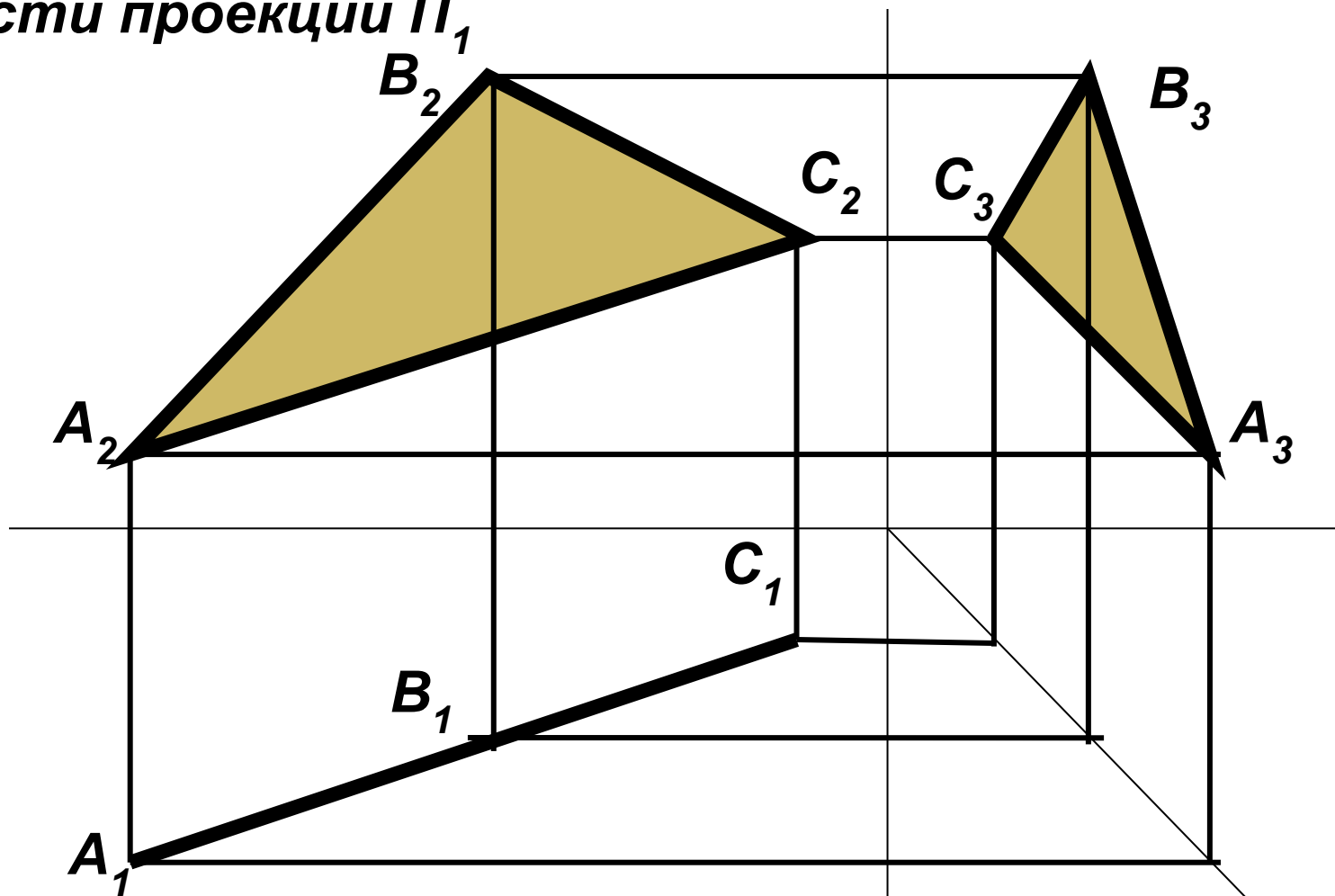
Чертеж горизонтально-проецирующей плоскости
