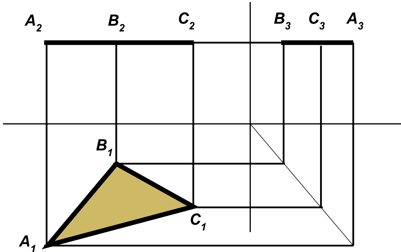
Чертеж горизонтальной плоскости уровня
