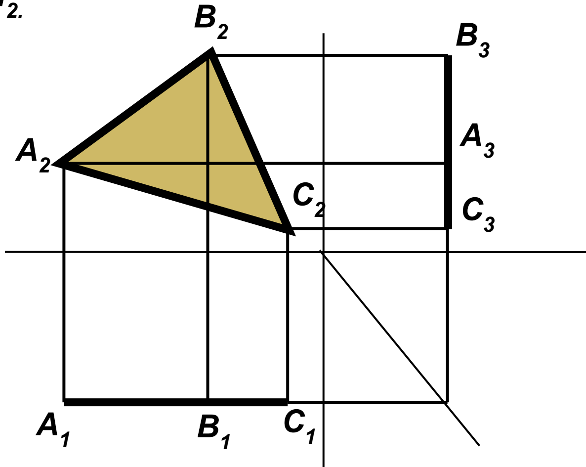
Чертеж фронтальной плоскости уровня
