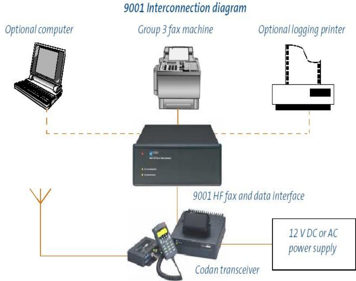
схема факсимільного зв'язку
