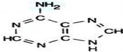
аденин (Ade)
