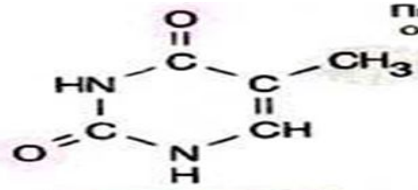
тимин (Thy)
