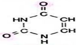
урацил (Ura)
