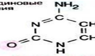
цитозин (Cyt)
