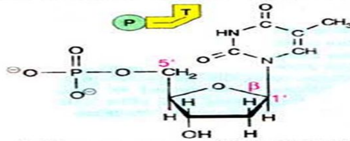
2. Дезокситимидин-5-фосфат (dTMP)
