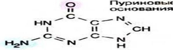
гуанин (Gua)
