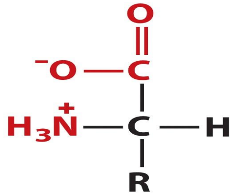
Цвиттерионная форма
