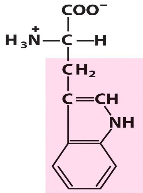
Триптофан (Trp)
