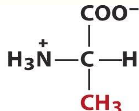
(c) L-Аланин
