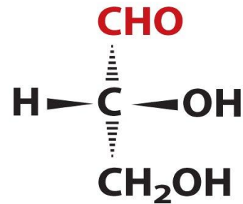
D-Глицеральдегид
