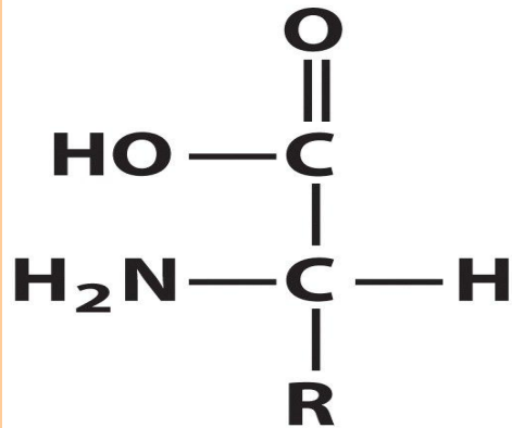
Нейтральная форма
