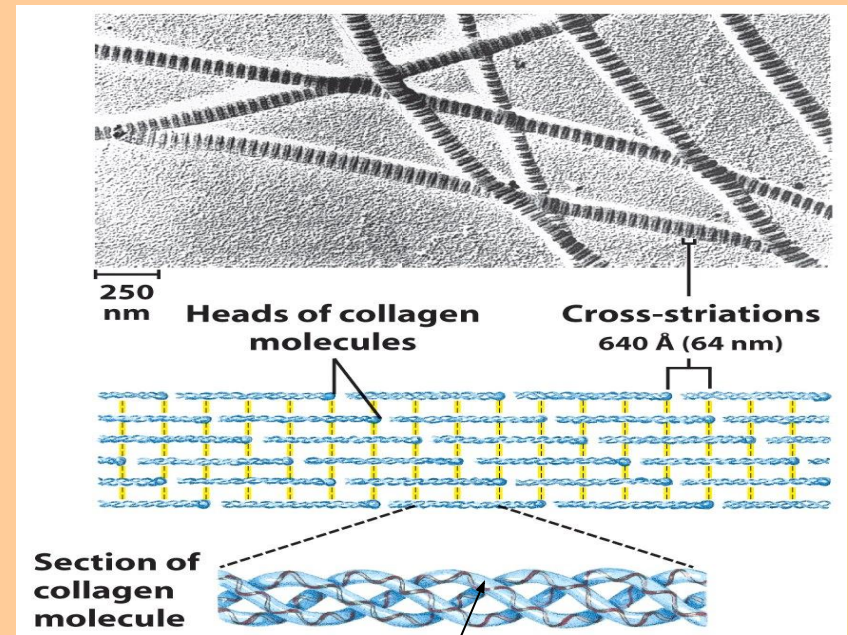
Тропоколлаген
