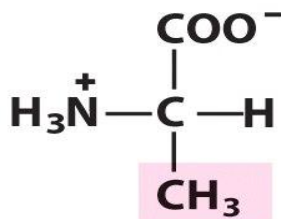
Аланин (Ala)
