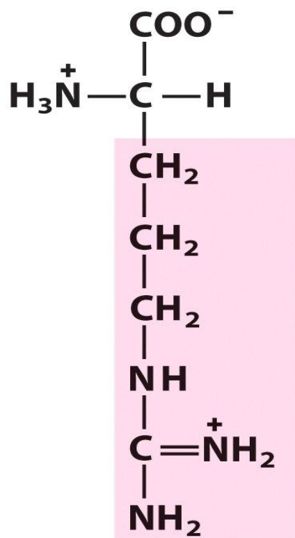
Аргинин (Arg)
