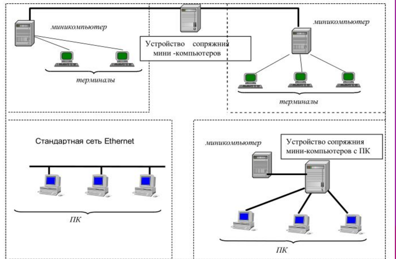
Рис. 1.5. Различные типы связей в первых локальных сетях
