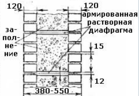
кладка с армированными растворными диафрагмами
