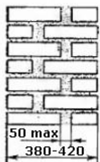
поперечные стенки с уширенными швами
