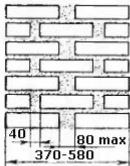
поперечные стенки с уширенными швами
