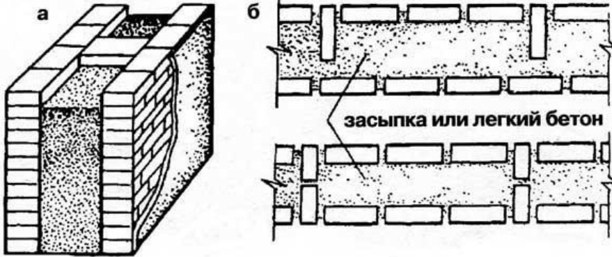
Колодцевая кладка с вертикальными поперечными стенами: а – общий вид; б – вид сверху
