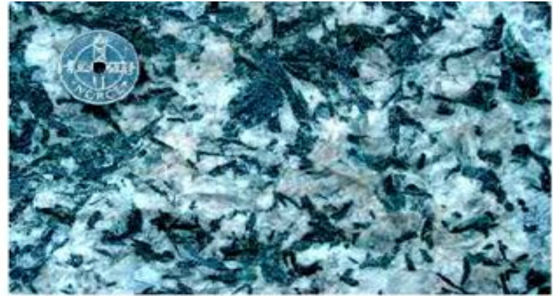
Роговая обманка и плагиоклаз
