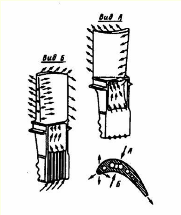
Рис. 1. Схема охлаждения лопатки газовой турбины авиационного двигателя
