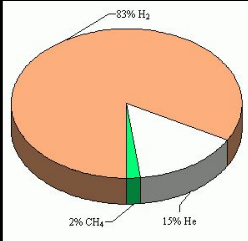
Химический состав атмосферы Урана
