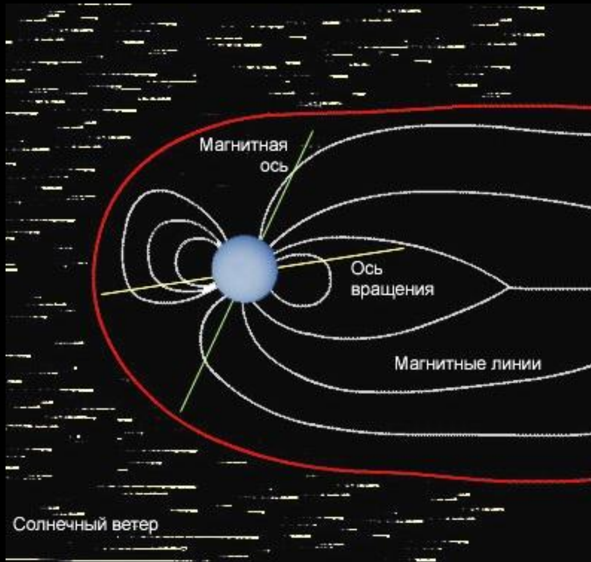
Магнитосфера Урана
