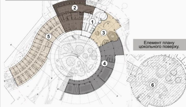
План першого поверху.
