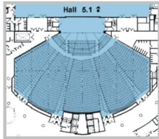
План зала "Гармония". Вариант трансформации
