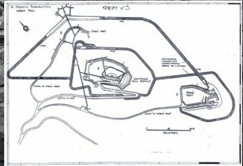
Схема из дипломного проекта по фортификации
