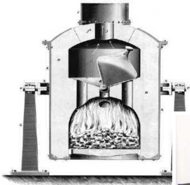
КОНВЕРТЕР (изобр. Г.Бессемер)
