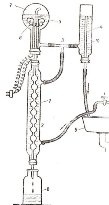
Дистилляция
