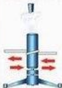
МЕХАНИЧЕСКАЯ РАБОТА
