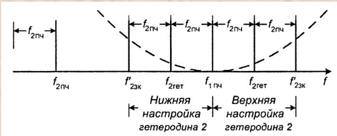
Рисунок 5 – расположение помехи по второму зеркальному каналу в тракте первой промежуточной частоты
