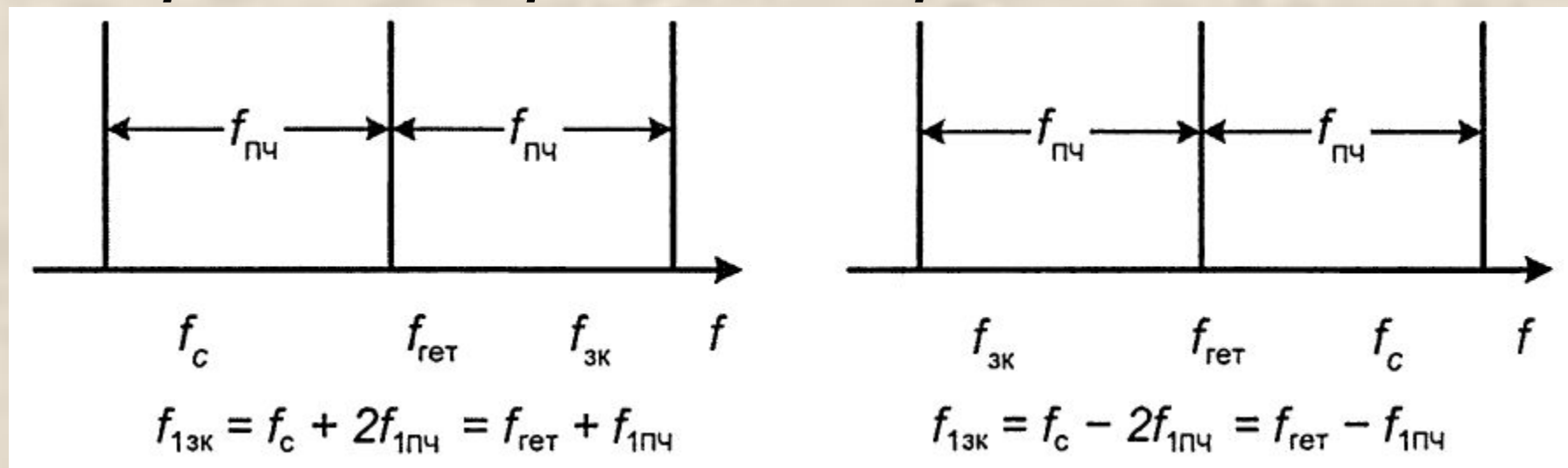
Рисунок 3 – Принцип образования помехи по первому зеркальному каналу
