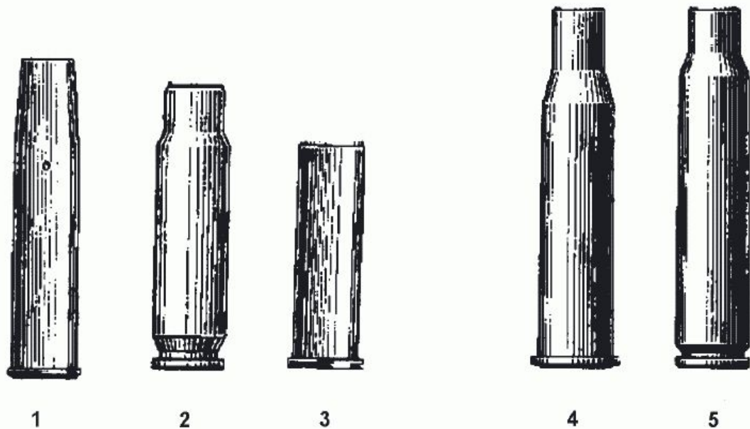
Рис. 2. Виды гильз по форме: 1 — коническая, 2 — бутылочная, 3 — цилиндрическая — и по устройству: 4 — с выступающим фланцем, 5 — с невыступающим фланцем
