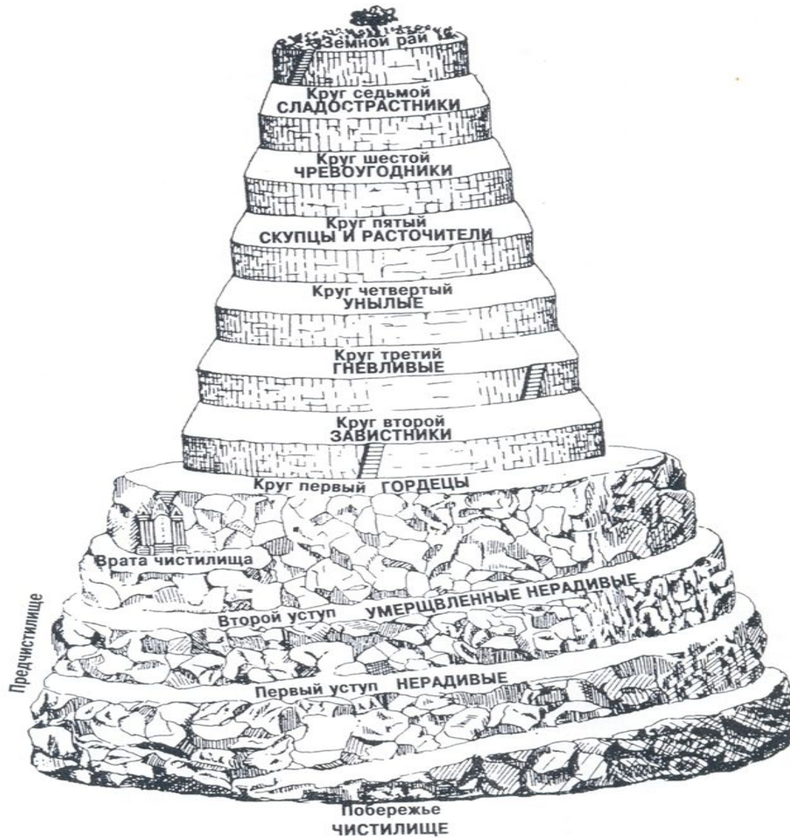
Схема Чистилища.
