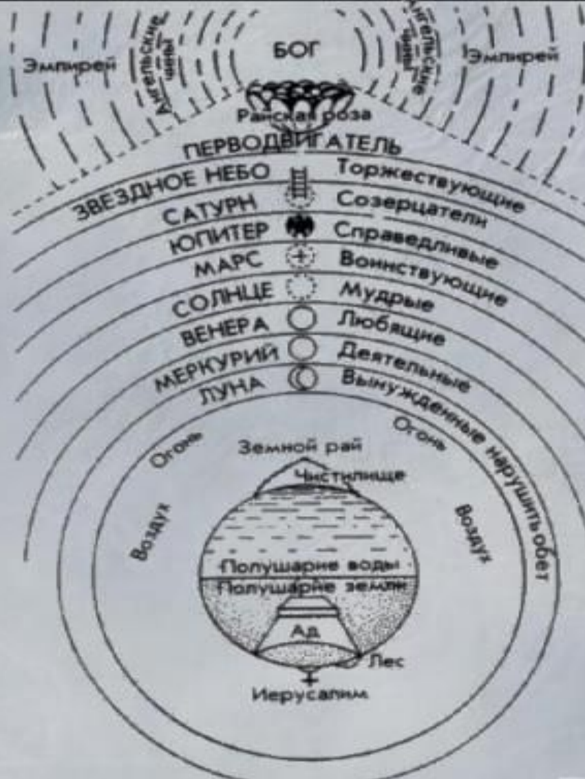
КОСМОС ДАНТЕ
