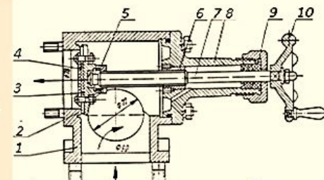
1 – корпус; 2 – седло клапана; 3 – клапан в сборе; 4 – прокладка; 5 – полукольца; 6 – втулка; 7 – шпindel; 8 – корпус задвижки; 9 – колпачок; 10 – маховичок
