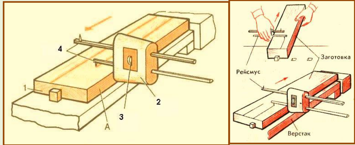
Рис. 2. Разметка рейсмусом: А – базовая кромка; 1- заготовка; 2 – колодка; 3 – клин; 4 – рейки с острыми шпильками.
