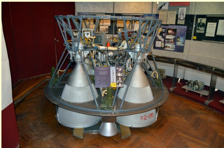
Ракетный двигатель РД 0110 воронежского производства
