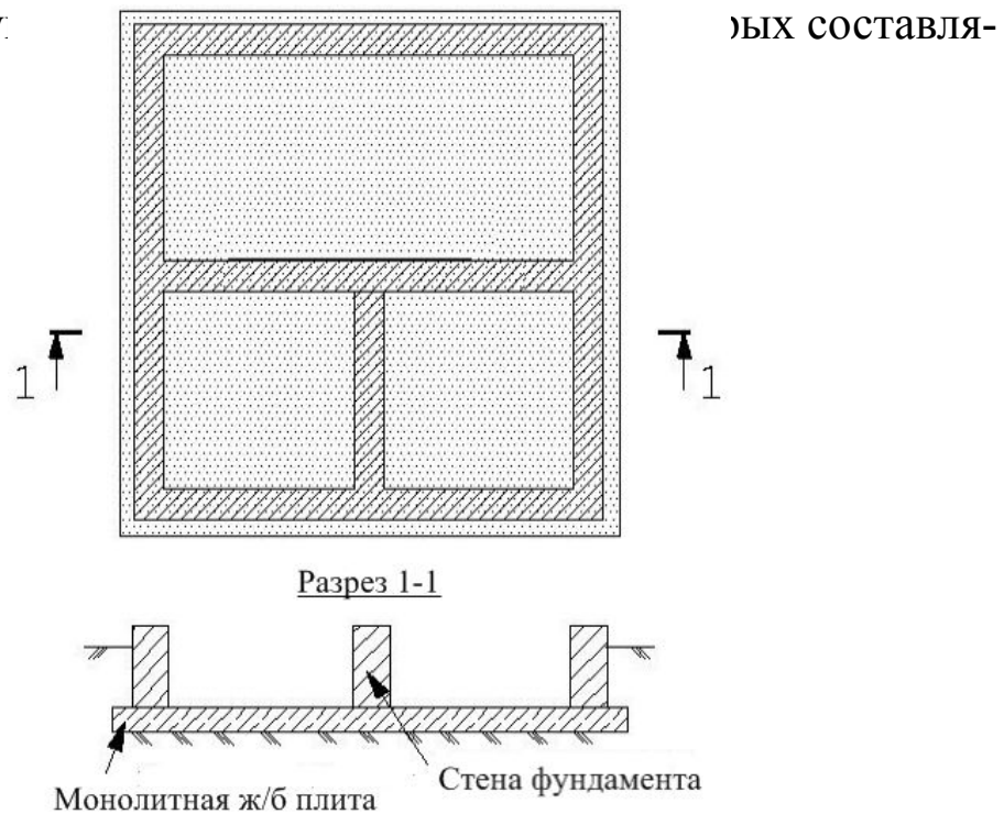
Устройство плитного фундамента
