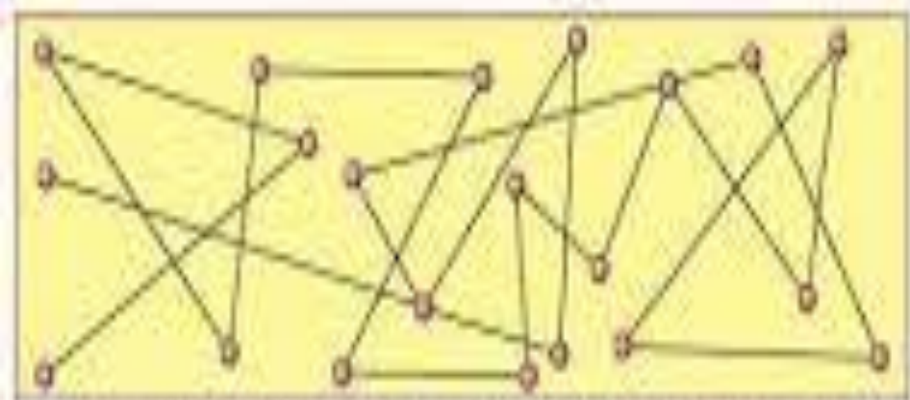
Подання траєкторії частинки через послідовні інтервали часу
