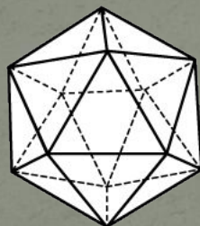
Икосаэдр {3,5}
