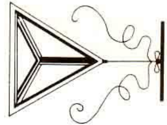
ТЕТРАЭДР
