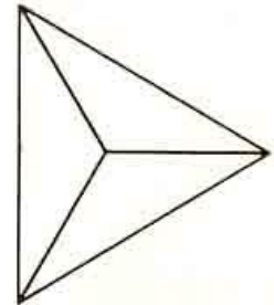
ТЕТРАЭДР
