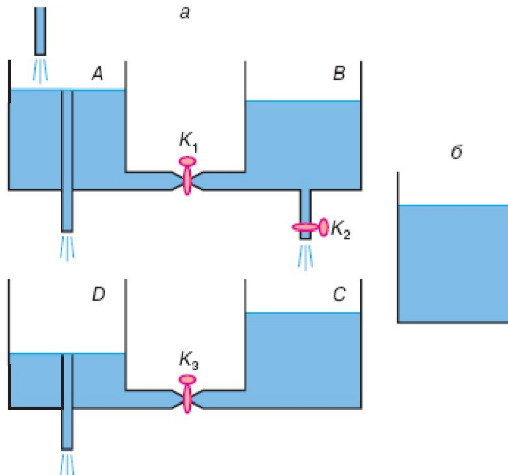
Рис. 2. Стационарное состояние. а – модель стационарного состояния (модель Бэртона). При определенной степени открытости кранов K_1 , K_2 и K_3 в баках В и С устанавливаются постоянные уровни, поскольку отток воды компенсируется ее притоком; б – постоянство уровня в непроточной емкости не является стационарным, так как не поддерживается динамически. Оно соответствует термодинамическому равновесию
