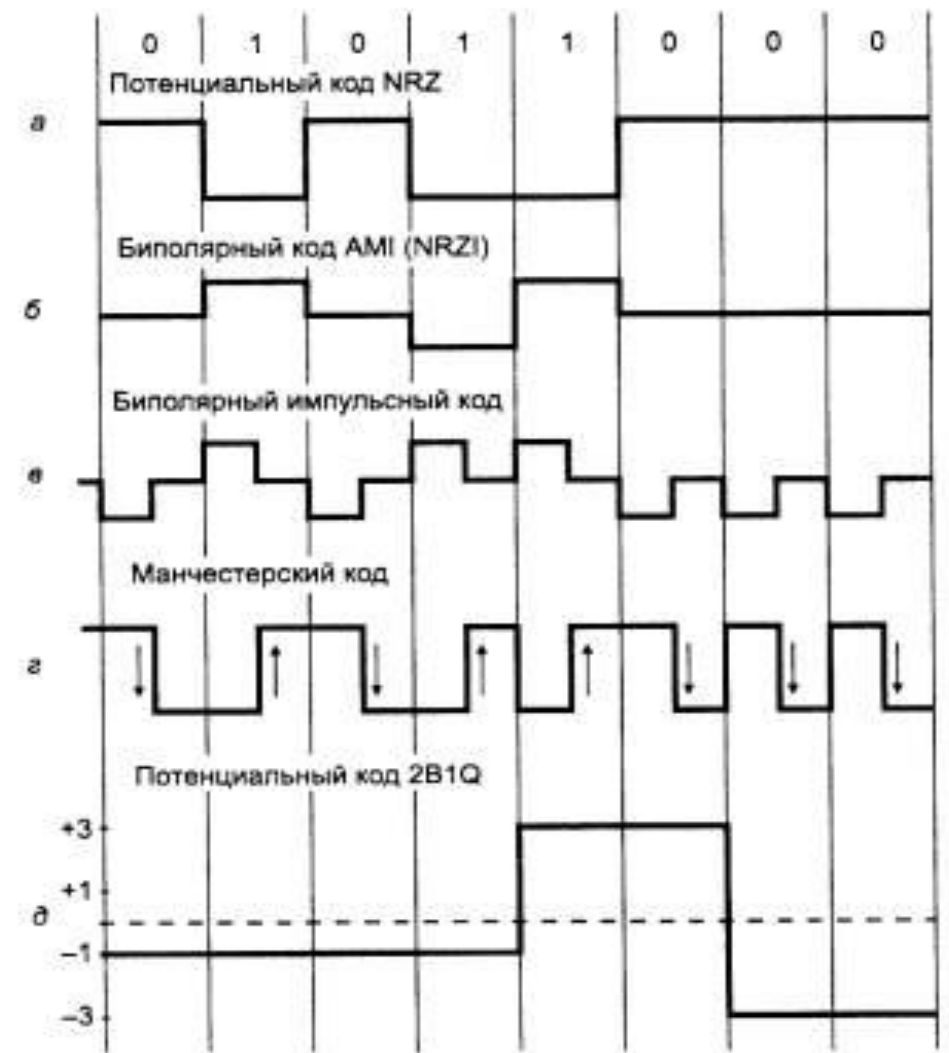
Рис. 5. Способы дискретного кодирования данных.
