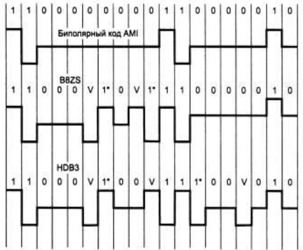
Рис. 6. Коды B8ZS и HDB3.
