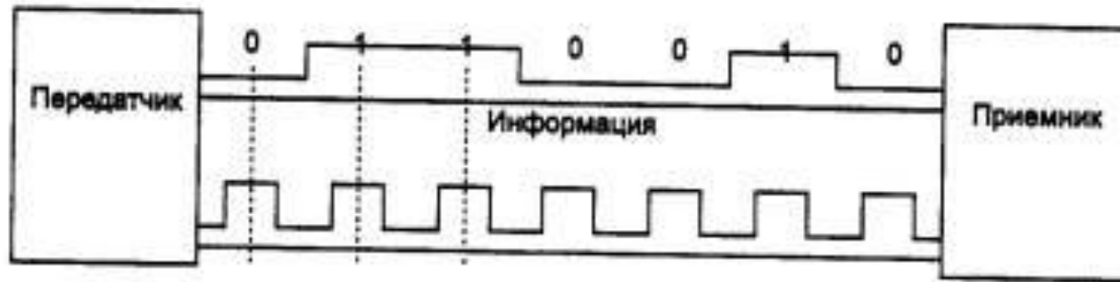
Рис. 4. Синхронизация приемника и передатчика на небольших расстояниях
