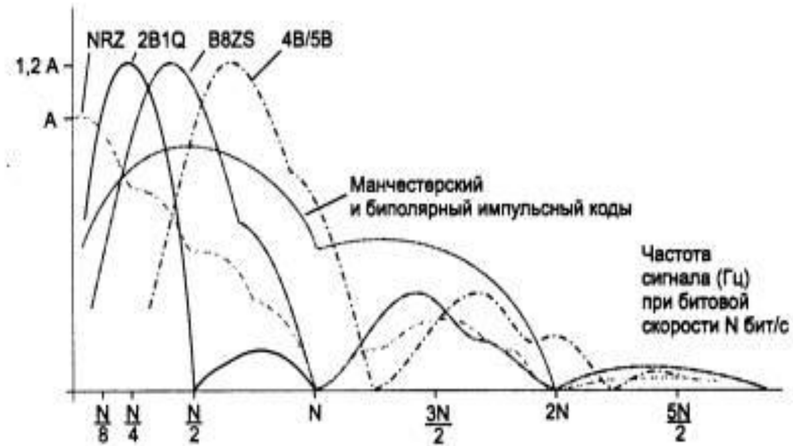
Рис. 7. Спектры потенциальных и импульсных кодов
