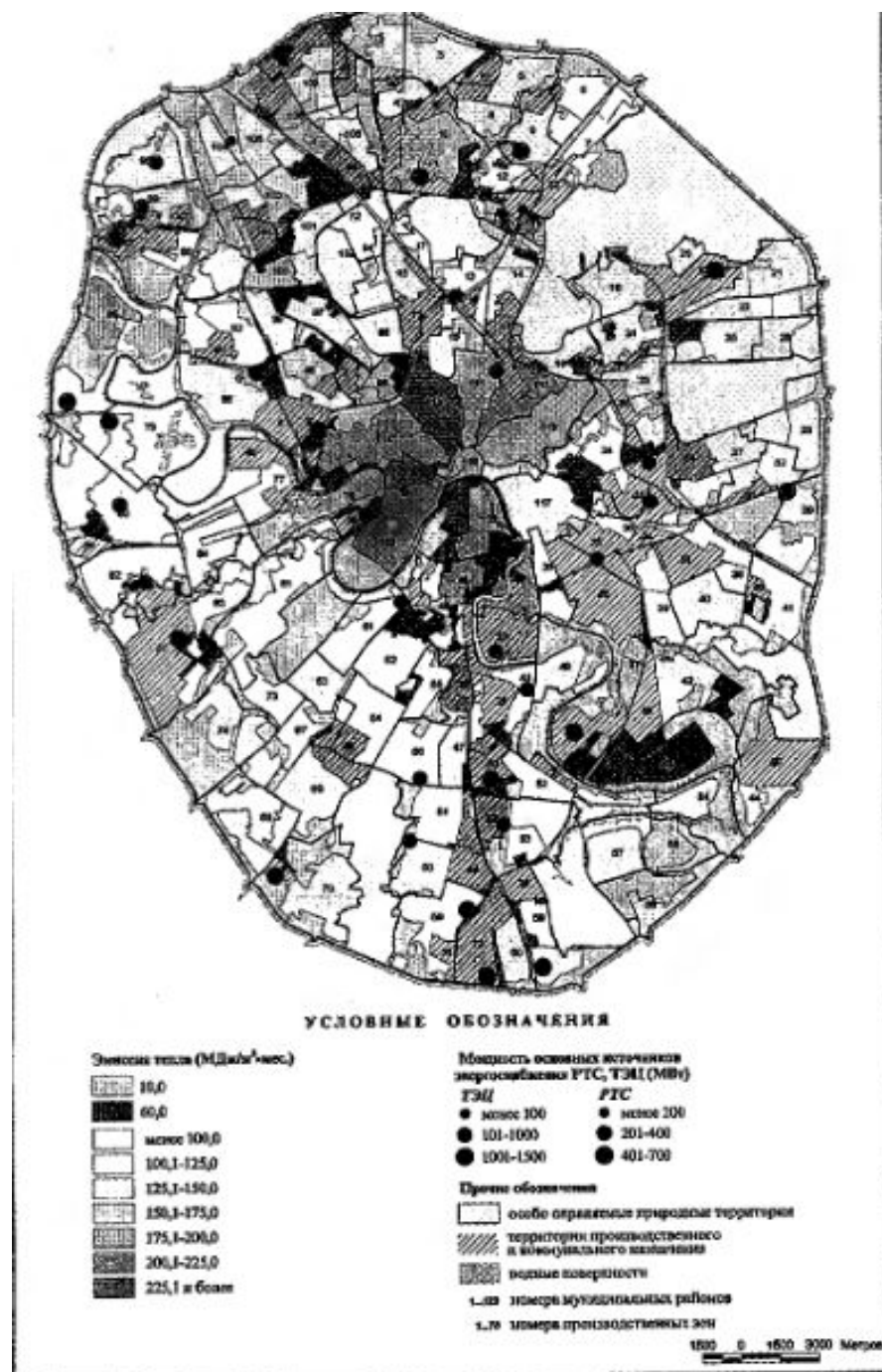
Рис. 3.10. Эмиссия техногенного тепла в окружающее пространство, январь
