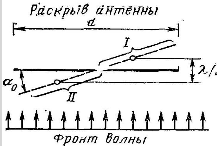
Рис. 4.31. Положение раскрытия антенны при максимальном и нулевом приеме.
