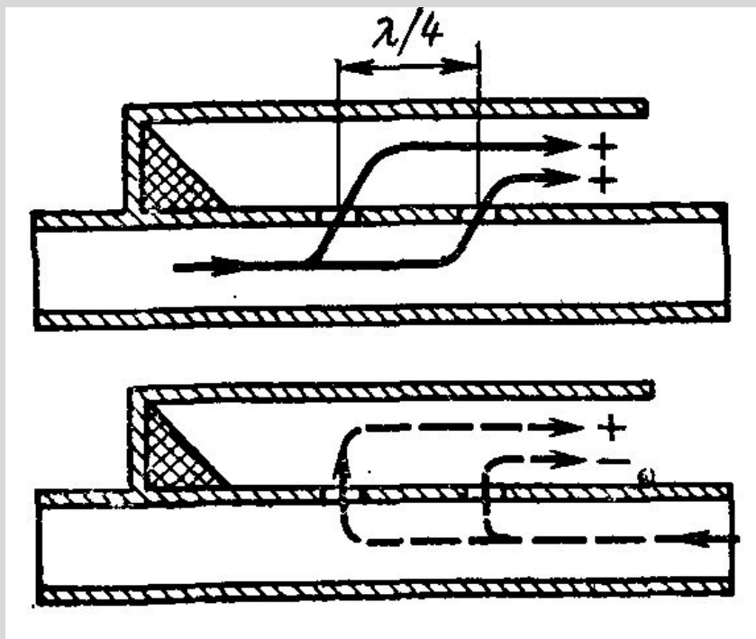
Рис. 4.23. Направленный ответвитель.
