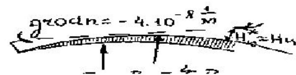
Рис.1.12. “Спрямление” луча при нормальной рефракции
