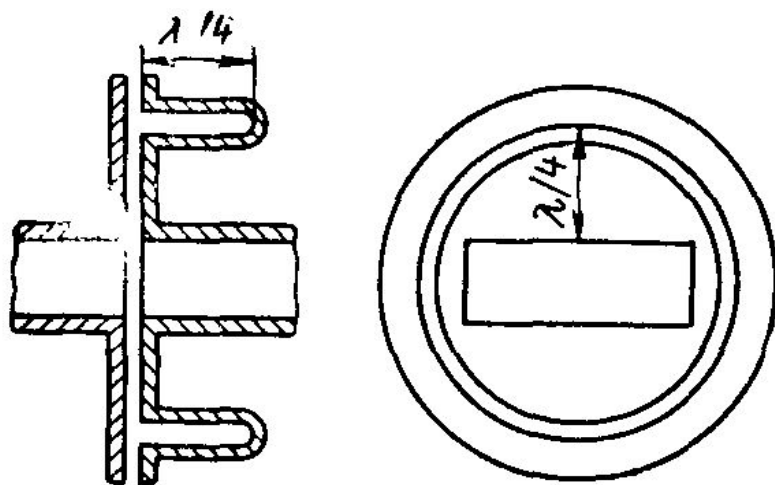
Рис. 4.21. Соединительный фланец волновода.
