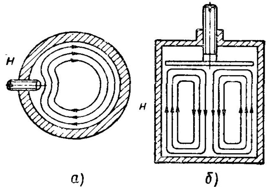
Рис. 4.18. Органы перестройки объемных резонаторов: винт (а), плунжер (б).
