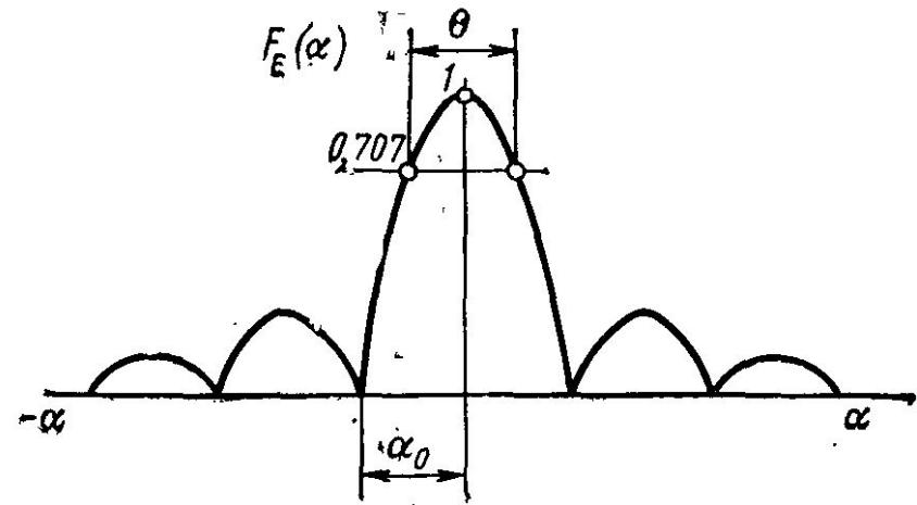
Рис. 4.32. Диаграмма направленности антенны по напряженности поля.
