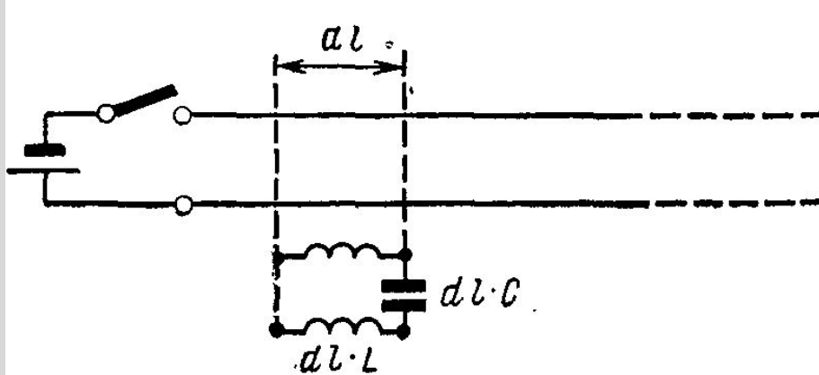
Рис. 3.15. Длинная линия и эквивалентная схема ее элемента.
