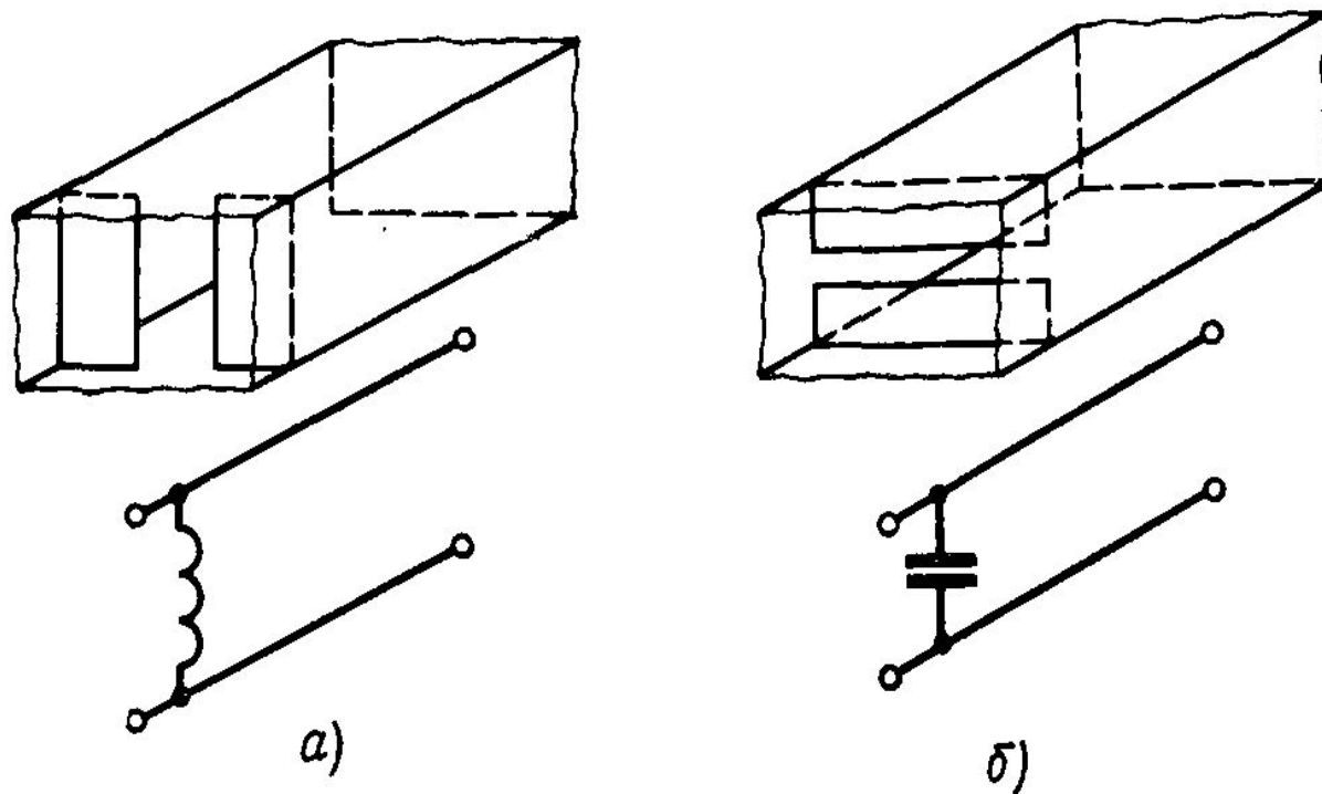
Рис. 4.16. Индуктивное (а) и емкостное (б) сопротивления в волноводе.
