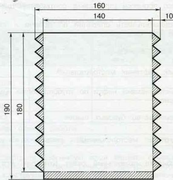
Развёртка цилиндра
