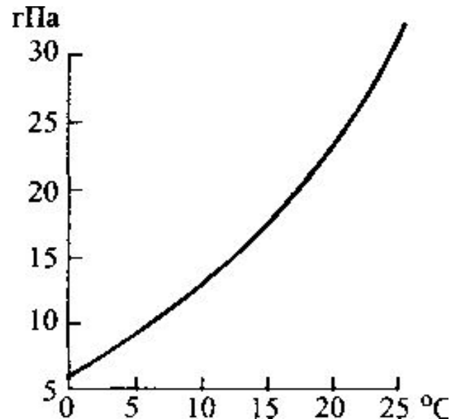
Рис. 1.5. Парциальное давление насыщенного водяного пара в зависимости от температуры
